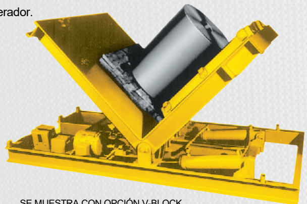
SE MUESTRA CON OPCIÓN V-BLOCK
