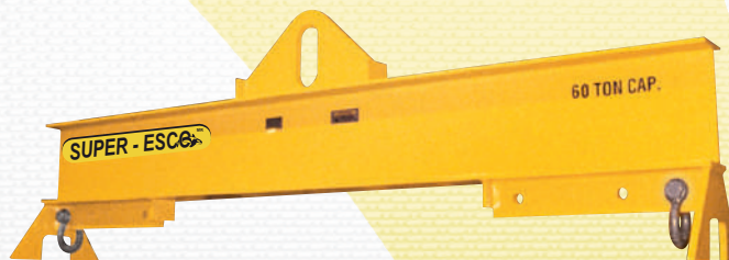
Aparece con soporte opcional sobre banco y diferente ubicación de los agujeros.
